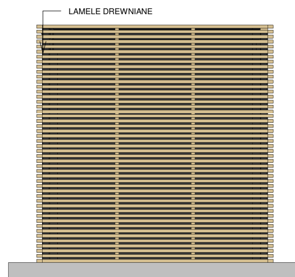
ELEWACJA WSCHODNIA
